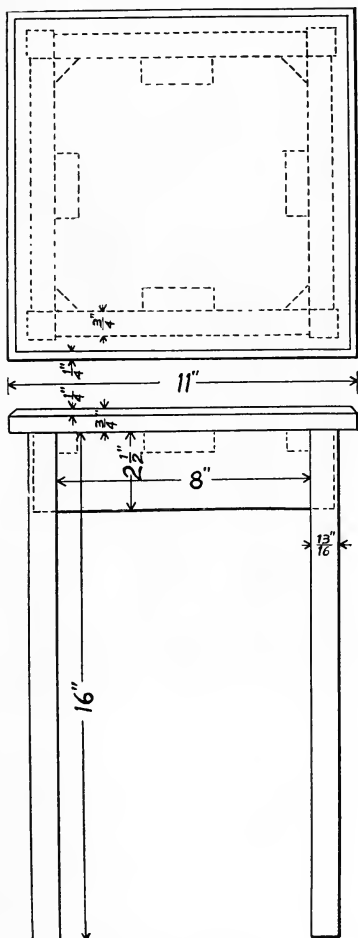
Fig. 181—Taboret
